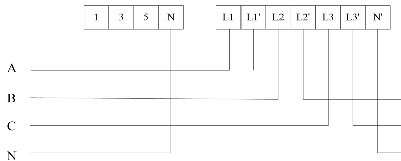
三相四线直接接入
