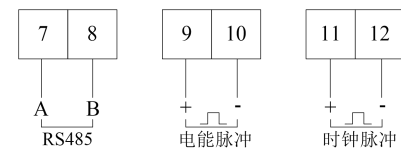
通讯及脉冲输出端子
